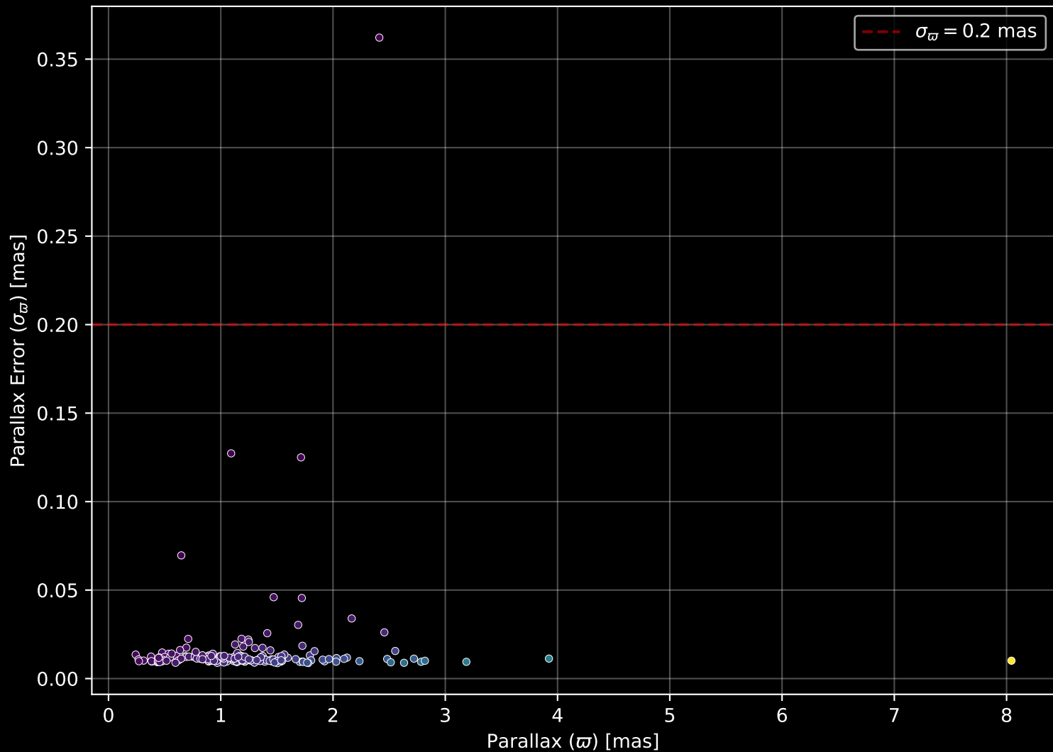
GALAH DR4 Field: [529] Parallax Quality (n= 187)
