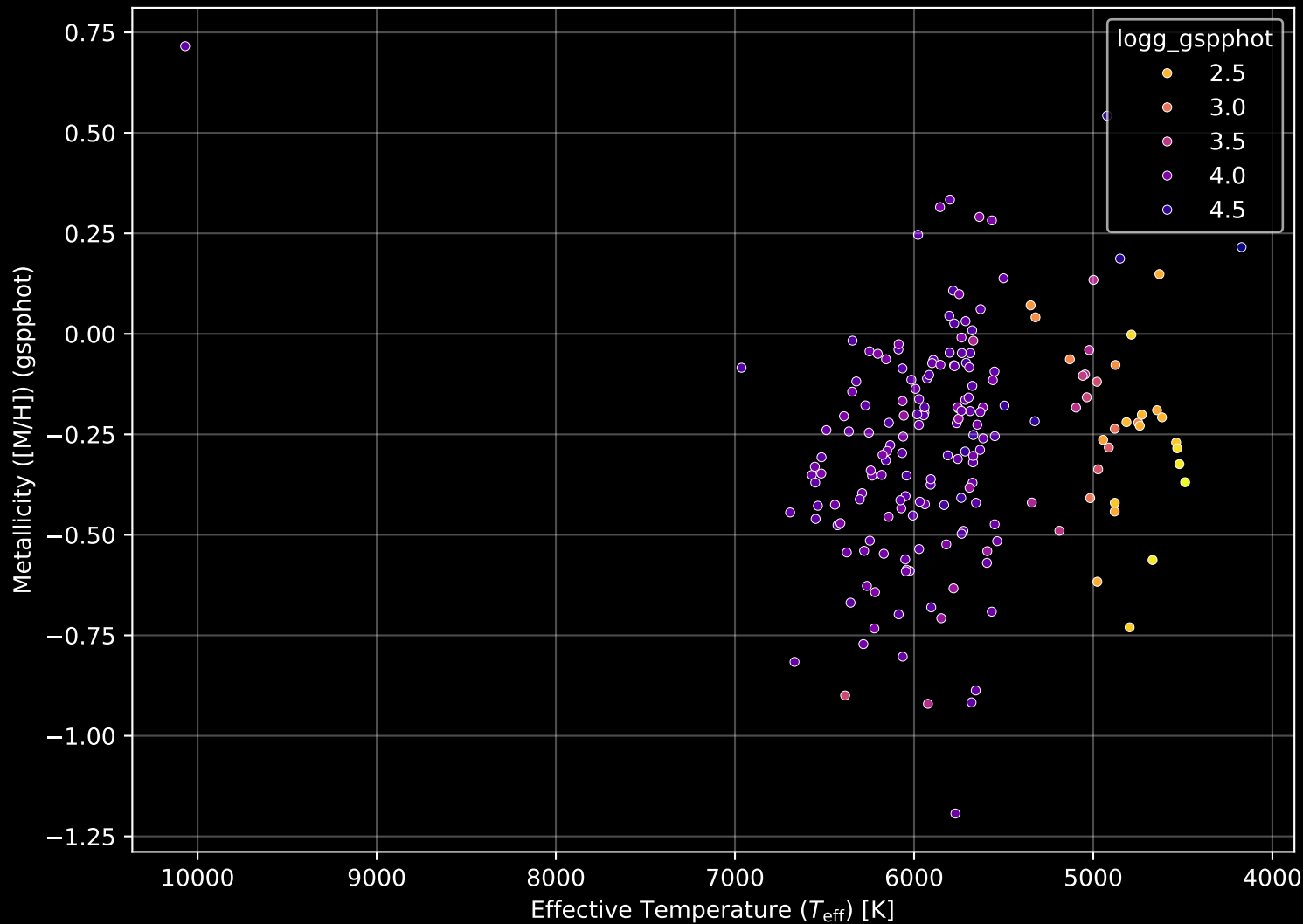
GALAH DR4 Field: [529] Stellar Population Parameters (n= 187)
